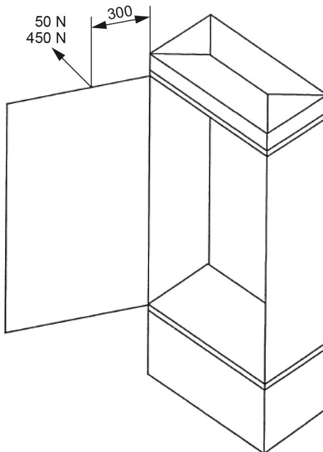
Obrázek 107 – Schematické znázornění zkoušky pro ověření mechanické pevnosti dveří
