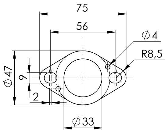
Flange 45E Cod.205267
